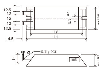
BB IRH200L~IRH500L
